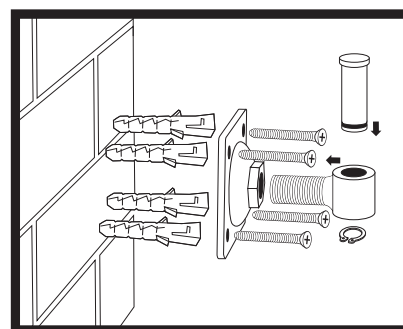
Blacha z nakrętką 80 x 80 mm Ø16 mm
