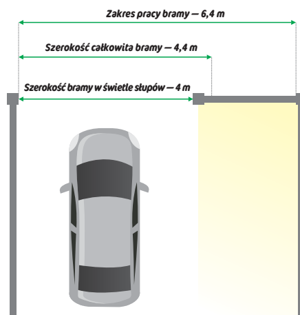
Brama segmentowa
